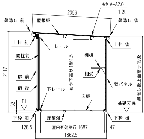
「物置部」矩計図 (S=1/50) ※<>内は積雪型を示す。
