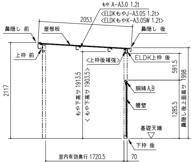
「オープン部」矩計図 (S=1/50) ※<>内は積雪型を示す。
