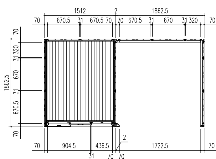
平面図 (s = 1/50)
