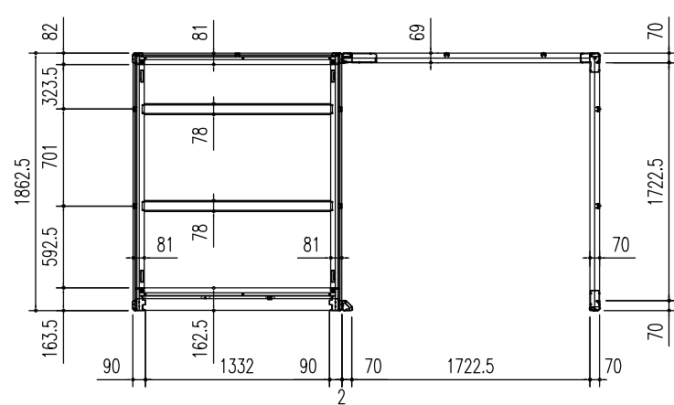
床伏図 (s = 1/50)
