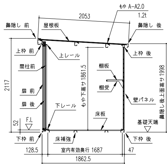
[物置部] 矩計図 (s = 1/50)
