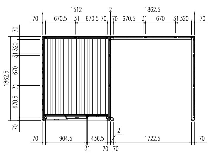
平面図 (s = 1/50)
