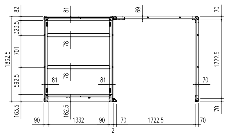
床伏図 (s = 1/50)
