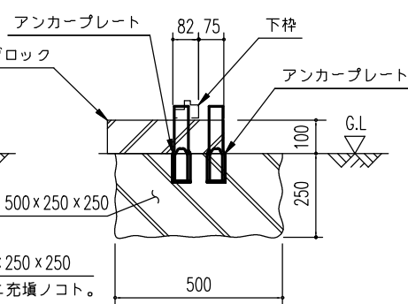
D ~ D' 断面 (外アンカー用)
