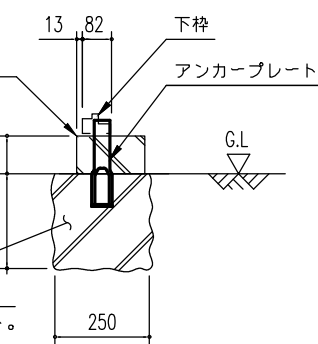
B ~ B' 断面 (外アンカー用)
