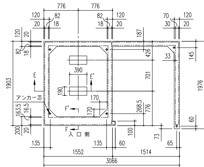
布基礎伏図 (S=1/50)
