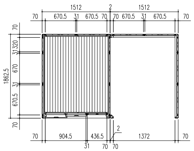
平面図 (S = 1/50)
