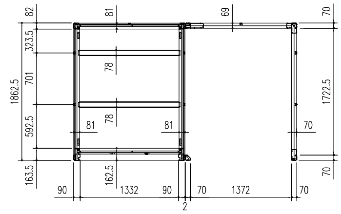
床伏図 (S = 1/50)
