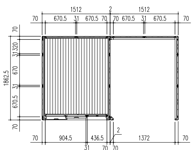
平面図 (S = 1/50)
