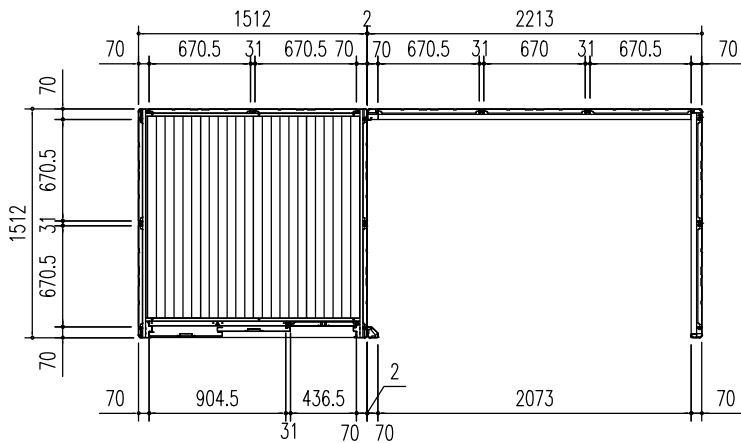
平面図 (s=1/50)
