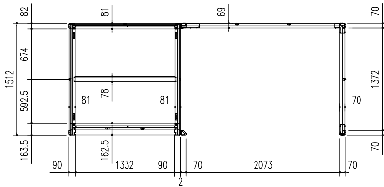
床伏図 (s=1/50)
