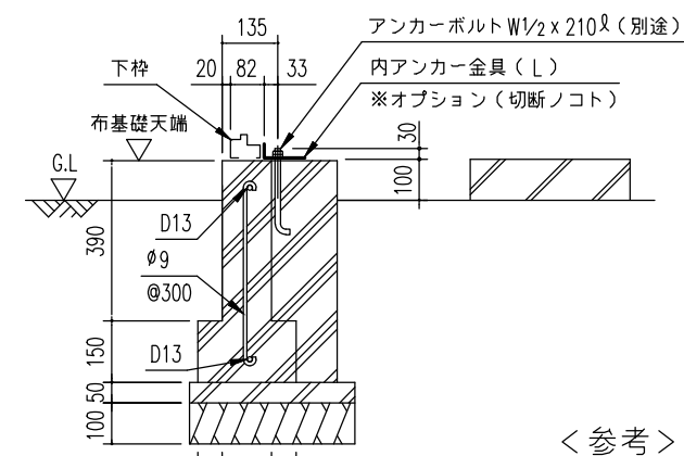
E ~ E' 断面
