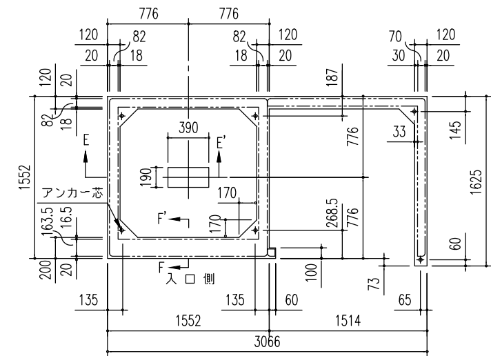
布基礎伏図 (S=1/50)
