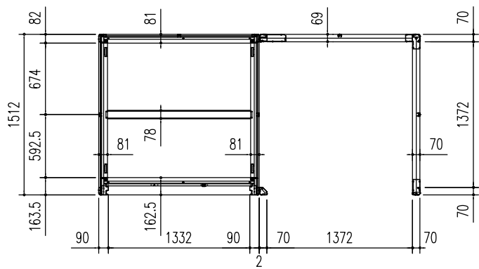
床 伏 図 (S = 1/50)
