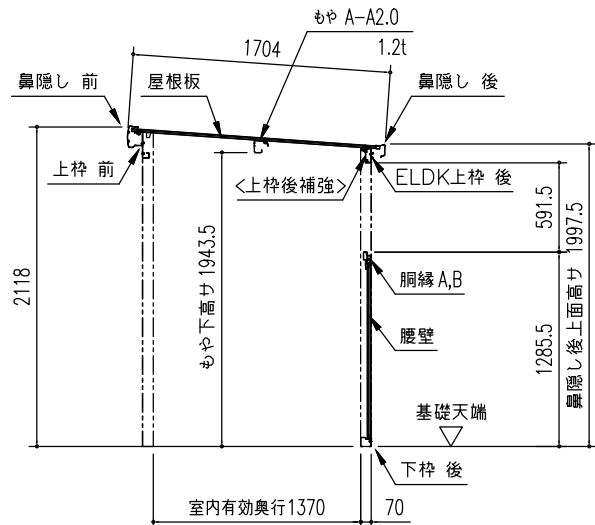
〔オープン部〕矩計図 (S = 1/50)
