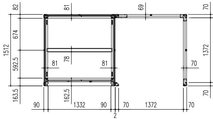
床伏図 (S = 1/50)
