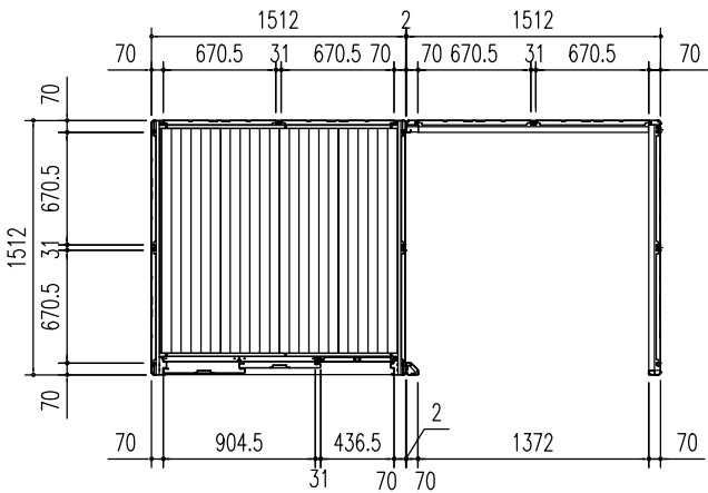
平面図 (S = 1/50)
