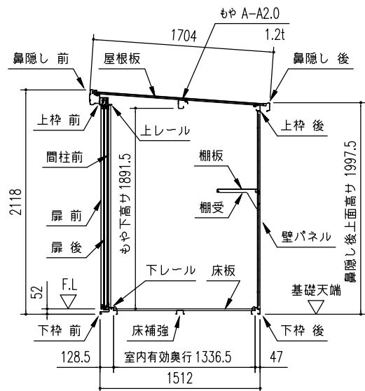
〔物置部〕矩計図 (S = 1/50)
