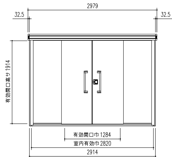
正面立面图 (S = 1/50)
