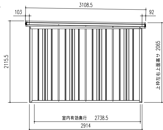
側面立面図 (S = 1/50)
