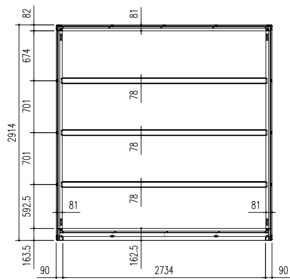
床 伏 図 (S = 1/50)
