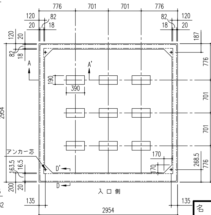
布基礎伏図 (S = 1/50)
