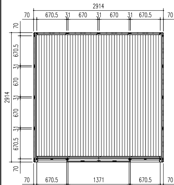
平面图 (S = 1/50)
