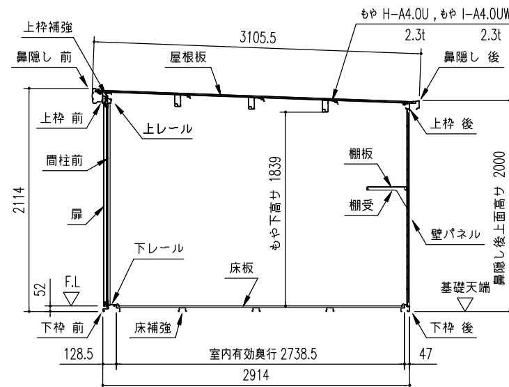
矩 計 図 (S = 1/50)
