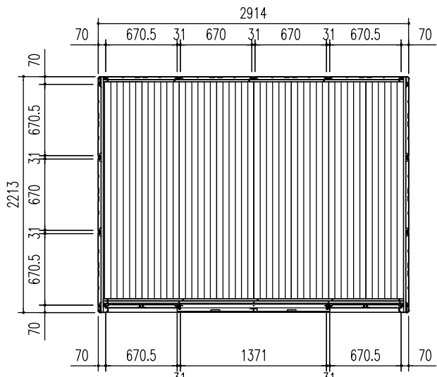
平面図 (S = 1/50)
