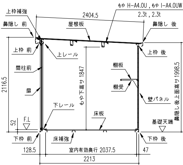
矩計図 (S = 1/50)
