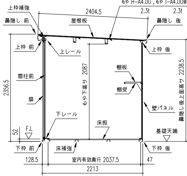
矩計図 (S = 1/50)
