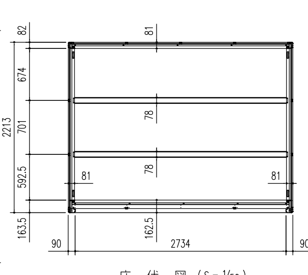
床 伏 図 (S = 1/50)
