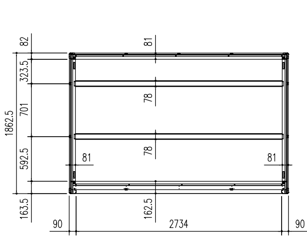
床 伏 図 (S = 1/50)
