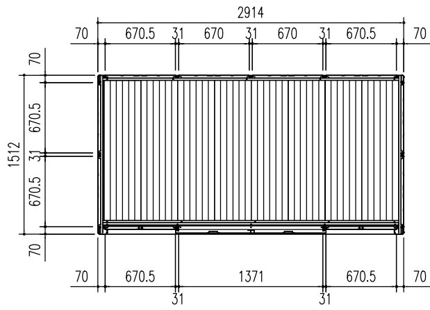
平面図 (S = 1/50)
