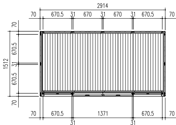
平面図 (S = 1/50)
