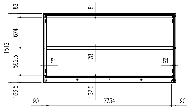
床 伏 図 (S = 1/50)
