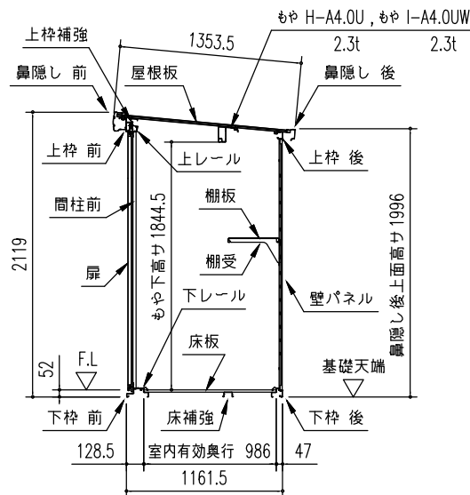
矩計図 (S=1/50)
