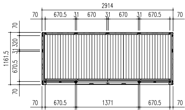
平面図 (S=1/50)
