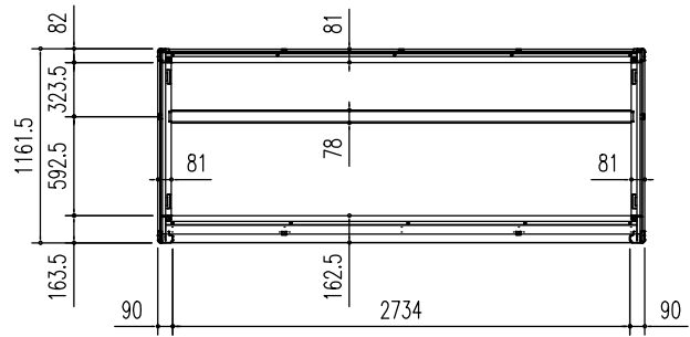
床 伏 図 (S=1/50)
