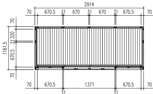
平 面 図 (S= 1/50)
