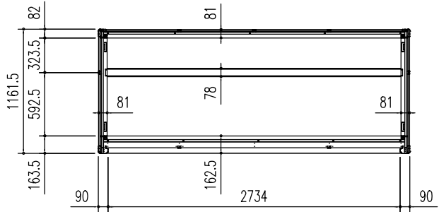
床 伏 図 (S= 1/50)
