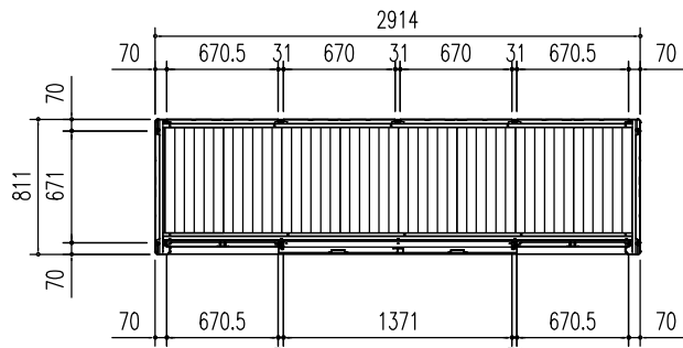
平面図 (S = 1/50)
