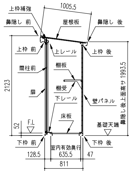
矩計図 (S = 1/50)
