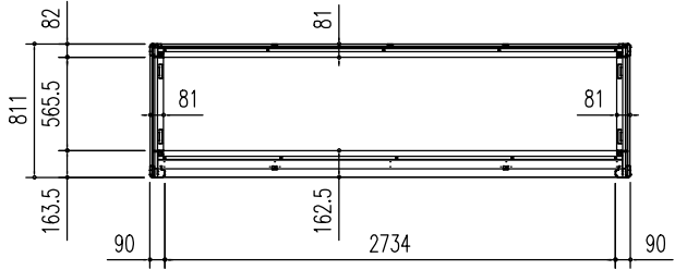
床 伏 図 (S = 1/50)
