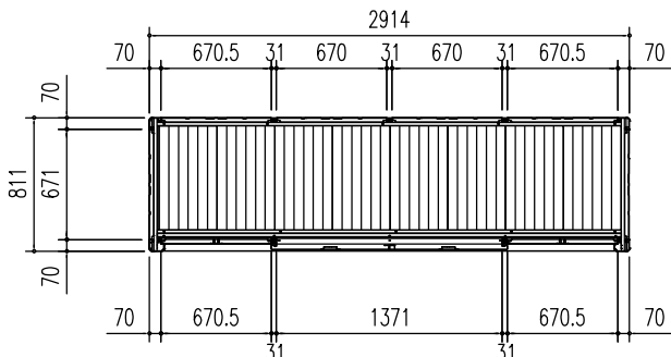
平面図 (S = 1/50)
