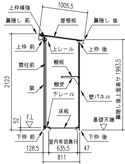
矩計図 (S = 1/50)
