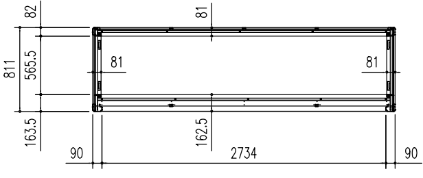
床 伏 図 (S = 1/50)
