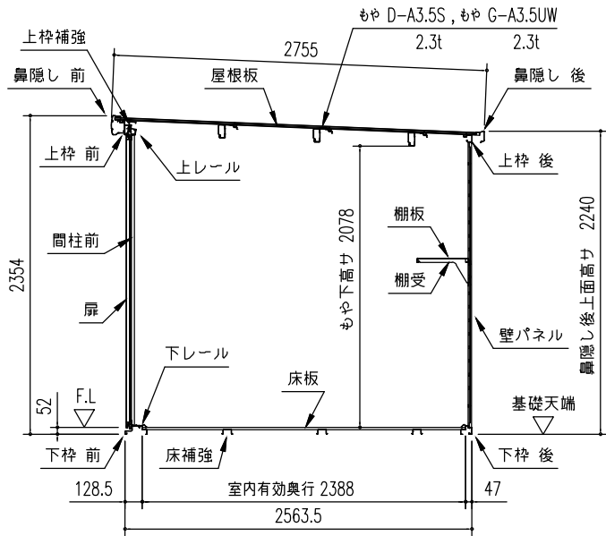
矩計図 (S = 1/50)
