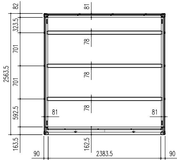
床伏図 (S = 1/50)
