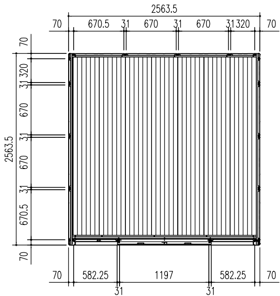
平面図 (S = 1/50)
