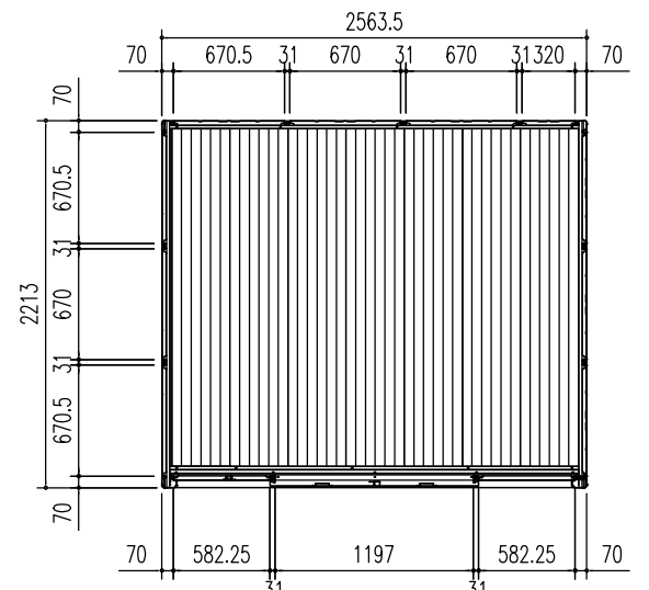
平面図 (S = 1/50)
