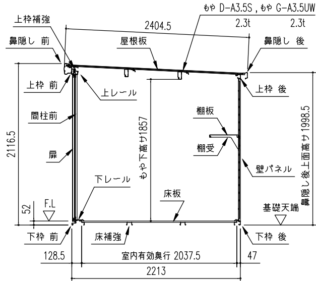
矩計図 (S = 1/50)
