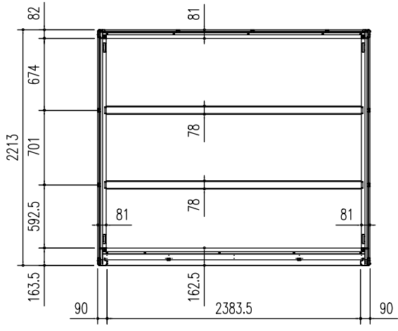
床伏図 (S = 1/50)
