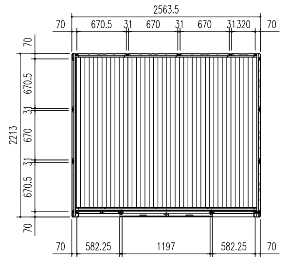
平面図 (S=1/50)
