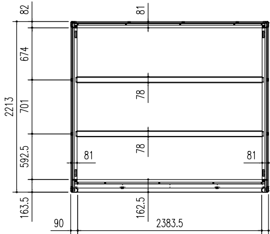
床伏図 (S=1/50)
