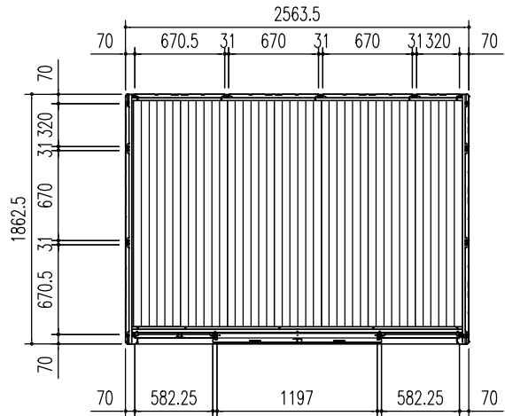
平面図 (S = 1/50)
