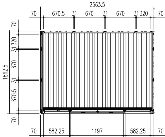
平面図 (S = 1/50)
