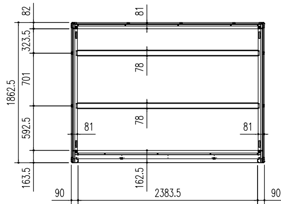
床 伏 図 (S = 1/50)
