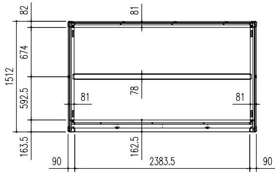
床 伏 図 (S = 1/50)
