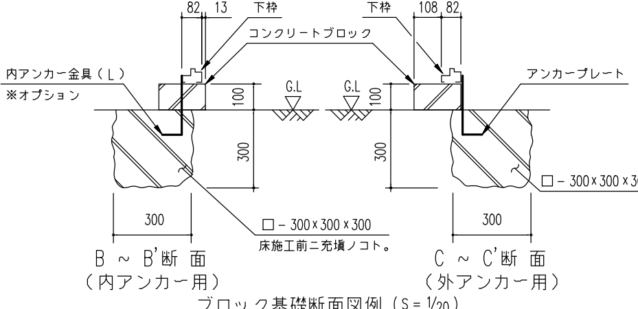
ブロック基礎断面図例 (S = 1/20)
