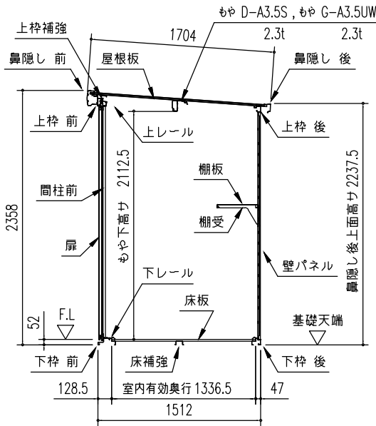
矩計図 (S = 1/50)
