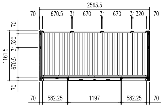
平面図 (S = 1/50)
