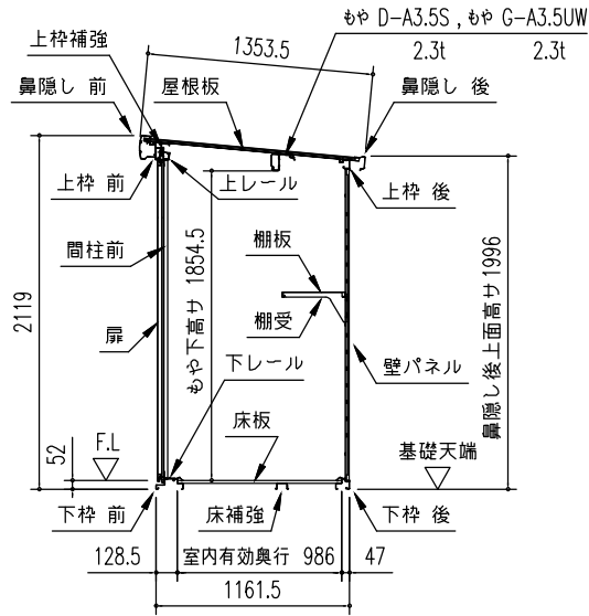
矩計図 (S = 1/50)
