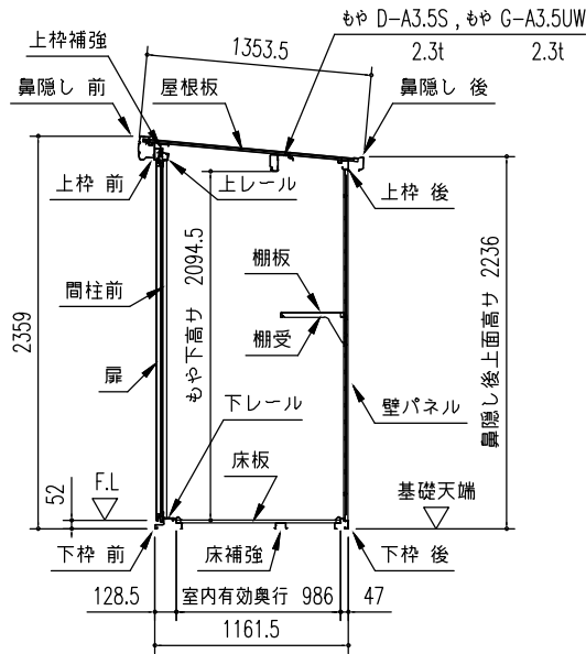
矩計図 (S = 1/50)
