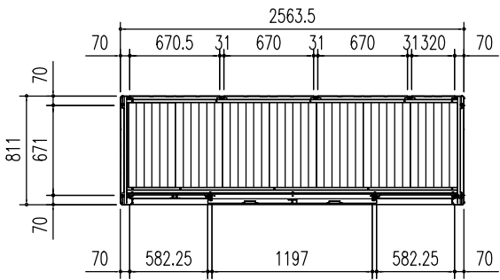
平面図 (S = 1/50)
