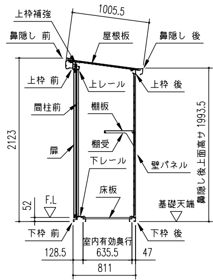
矩計図 (S = 1/50)
