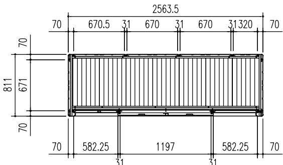
平面図 (S=1/50)
