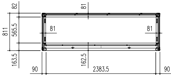
床 伏 図 (S=1/50)
