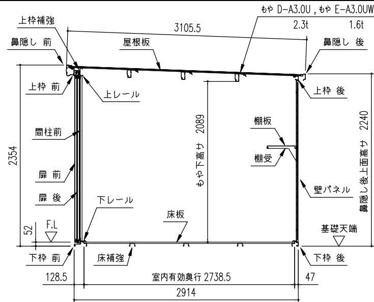
矩 計 図 ( S = 1/50 )
