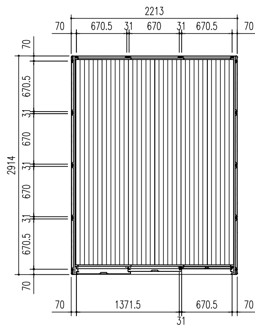
平面图 (S = 1/50)
