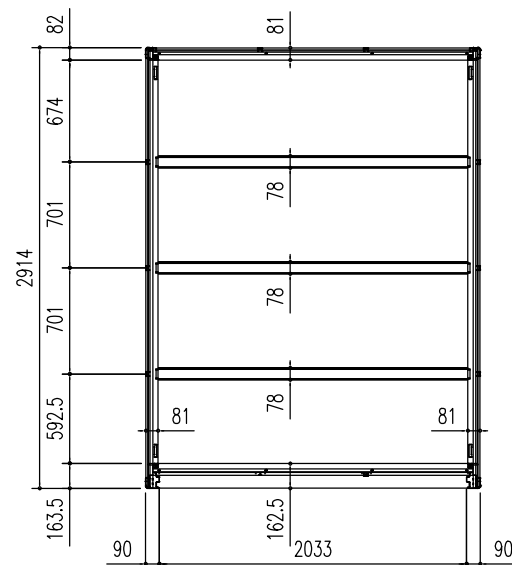
床 伏 図 (S = 1/50)
