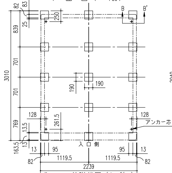
平面图 (S = 1/50)
