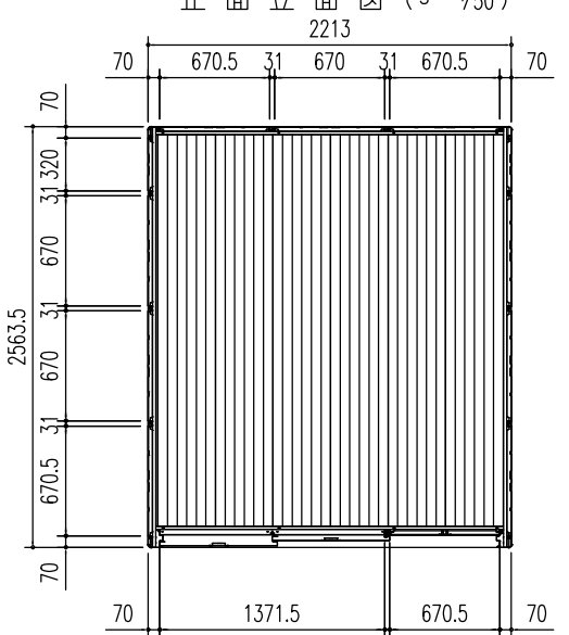
平面図 (S=1/50)
