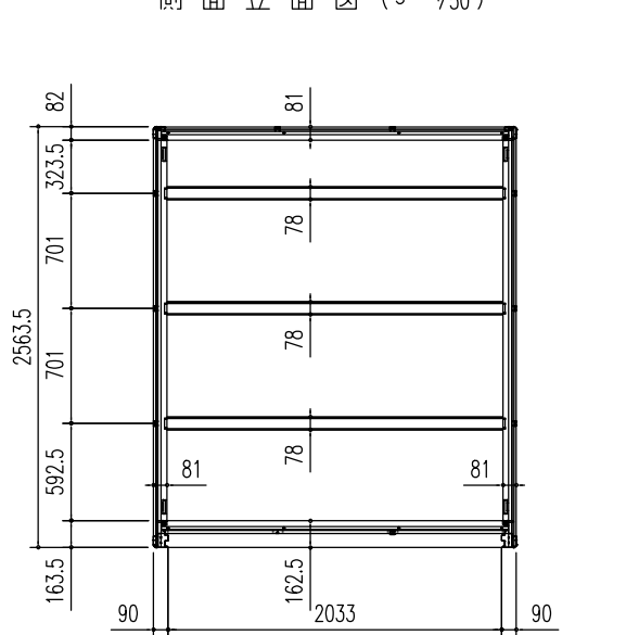
床伏図 (S=1/50)
