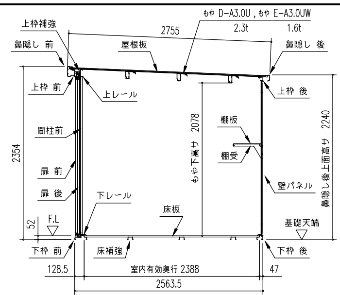
矩計図 (S=1/50)
