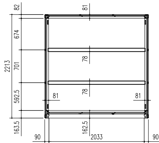
床 伏 図 (S = 1/50)
