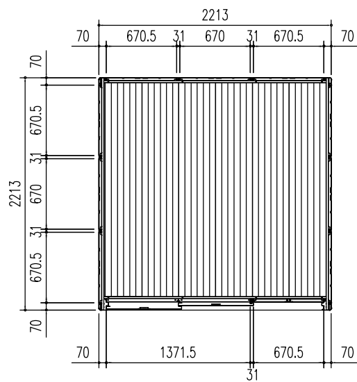
平面图 (S = 1/50)
