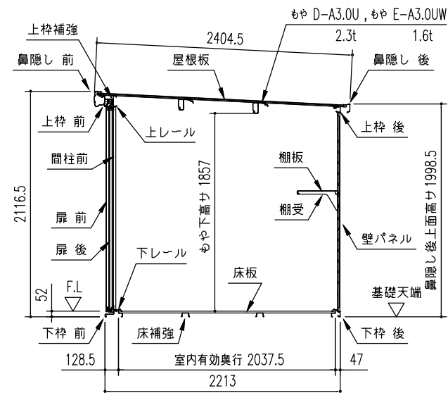
矩 計 図 (S = 1/50)
