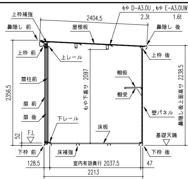
矩計図 (S=1/50)
