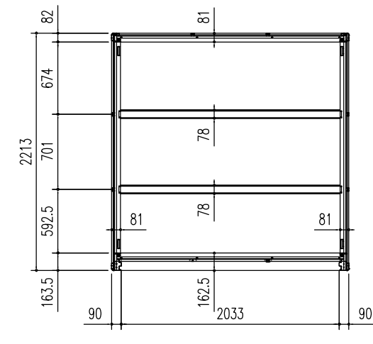
床伏図 (S=1/50)
