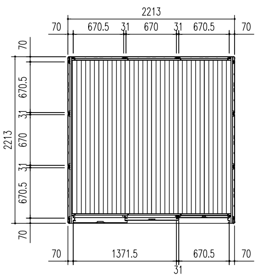
平面図 (S=1/50)
