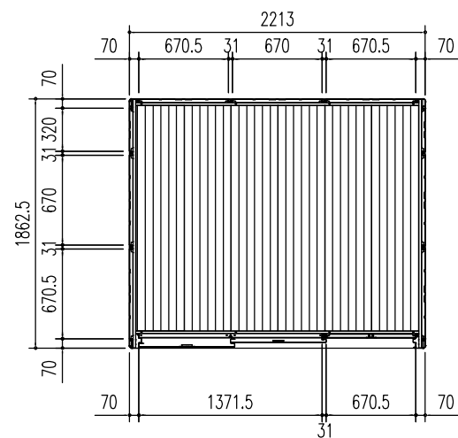
平面圖 (S = 1/50)
