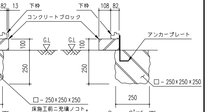
C ~ C' 断面 (外アンカー用)
