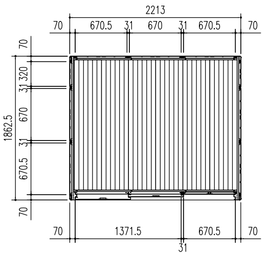
平面図 (S=1/50)
