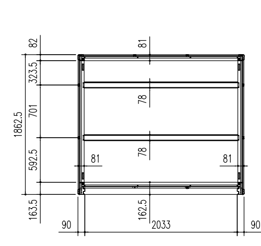
床伏図 (S=1/50)
