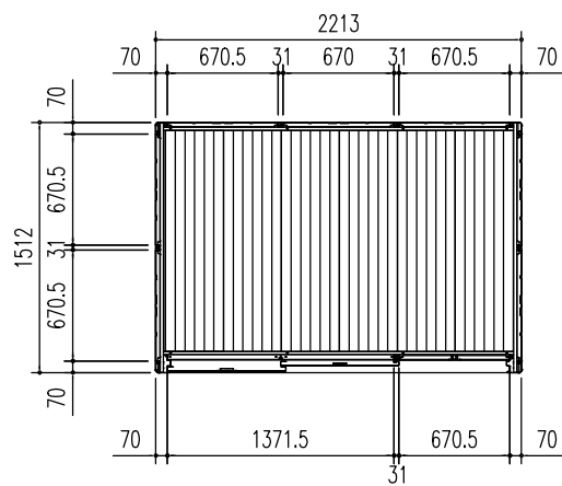
平面图 (S = 1/50)
