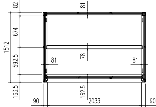
床伏図 (S=1/50)
