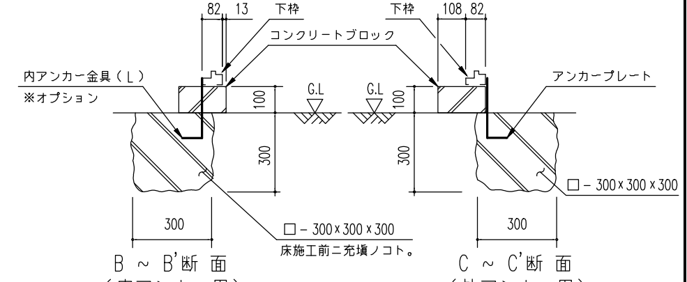
B ~ B'断面 (内アンカー用) C ~ C'断面 (外アンカー用)
