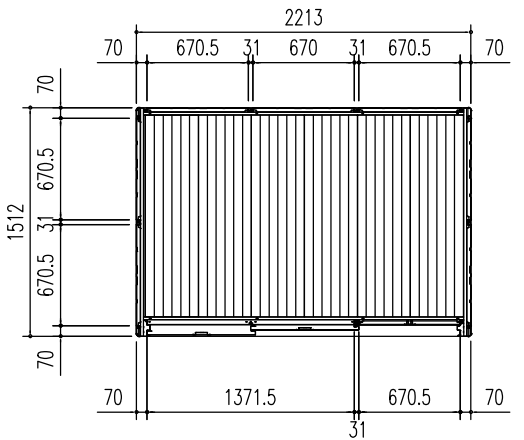
平面図 (S=1/50)
