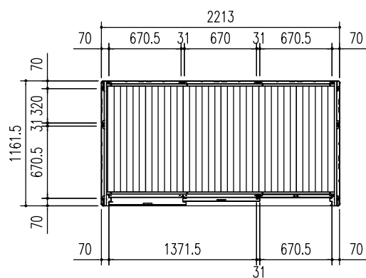
平面圖 (S = 1/50)
