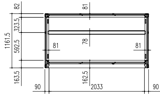
床伏図 (S=1/50)
