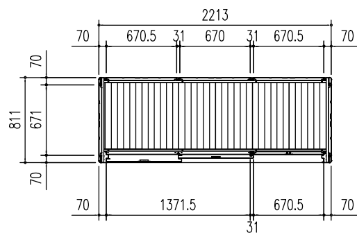
平面図 (S=1/50)
