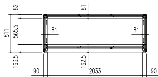
床 伏 図 (S=1/50)
