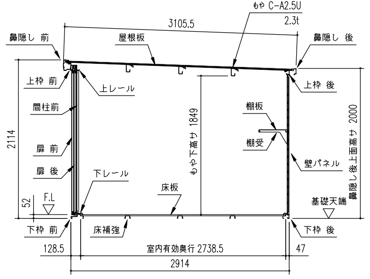
矩計図 (S=1/50)
