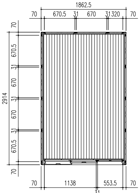
平面図 (S=1/50)
