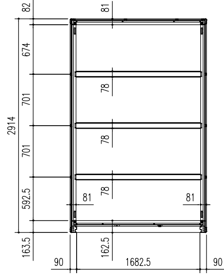
床伏図 (S=1/50)
