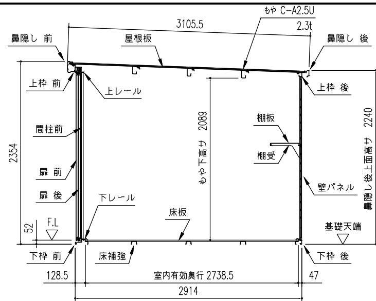
矩 計 図 ( S = 1/50 )
