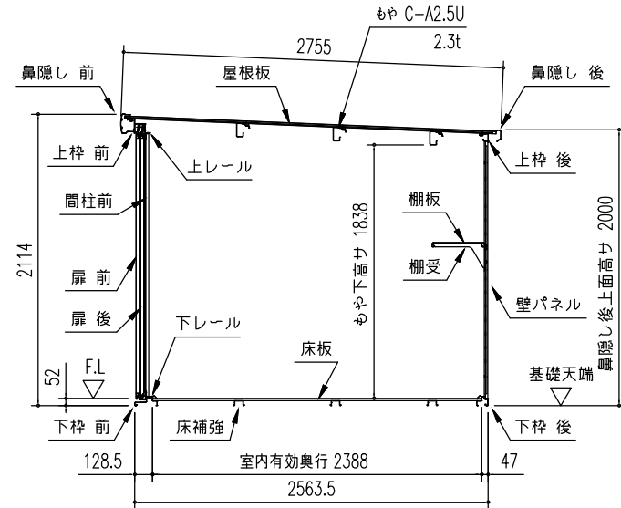
矩計図 (S=1/50)
