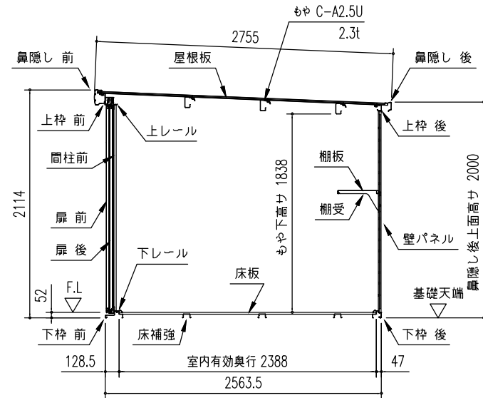
矩計図 (S=1/50)
