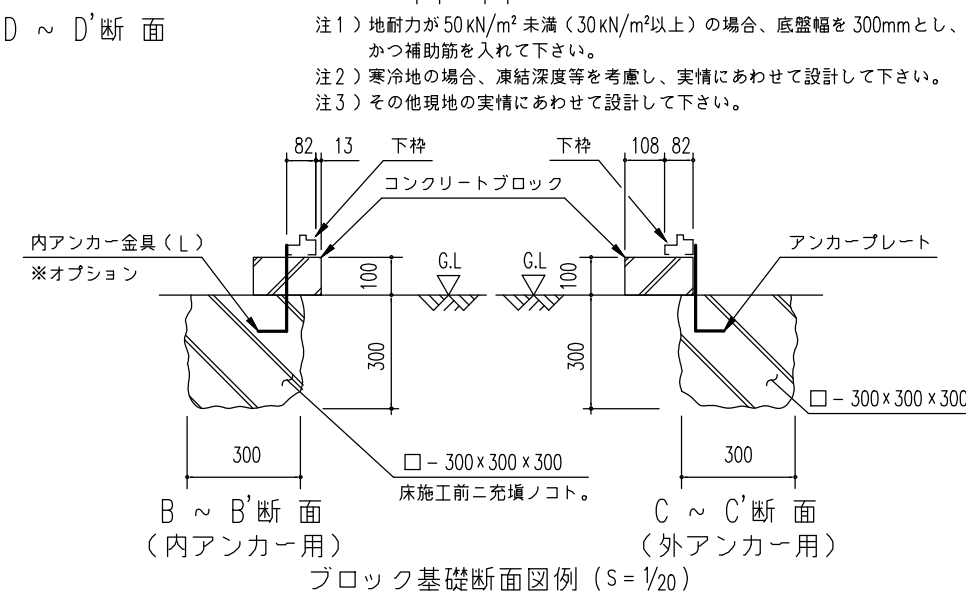
＜参考＞ (地耐力 50 kN/m 2 以上, コンクリート設計基準強度 18 N/mm 2 以上 基準風速 34 m/s, 地表面粗度区分Ⅲ) A ~ A' 断面 布基礎断面図例 (S = 1/20)
