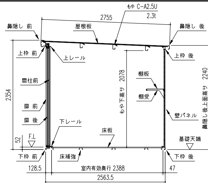
矩 計 図 ( S = 1/50 )
