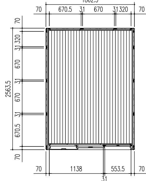
平面図 (S = 1/50)
