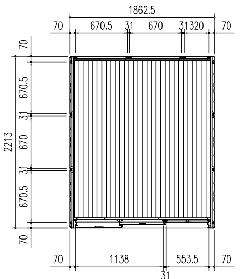
平面図 (S=1/50)
