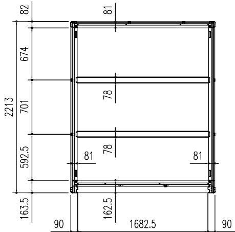
床伏図 (S=1/50)
